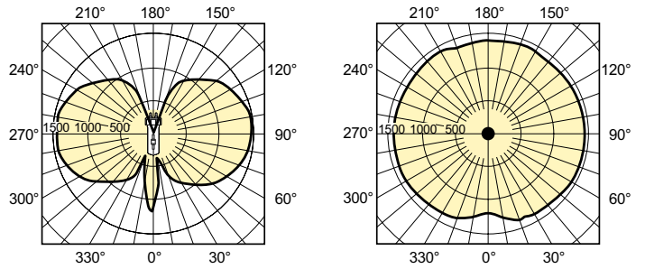
CDM-T 150W /830, /930, /942
