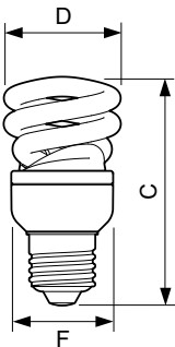
Twister 8W/827 E27 220-240V 50/60Hz
