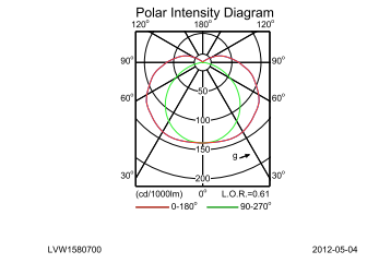
TCW060 2xTL-D18W HF
