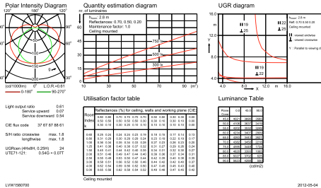
TCW060 2xTL-D18W HF
