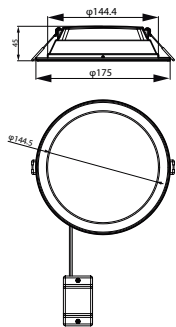
DN065B G4 LED12/830 12W 220-240V D150 RD
