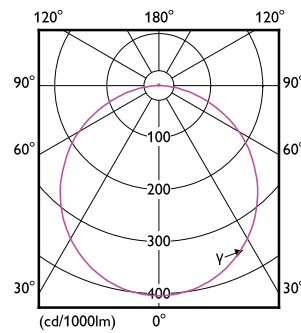
DN065B G4 LED12 830 12W D150 RD
