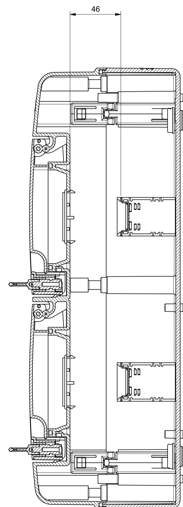
Sezione A-A
