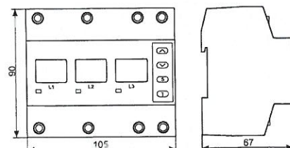
Dimensiuni de gabarit
