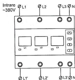
Schema de montaj
