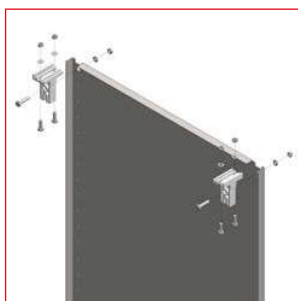
Montageplattenbefestigung
