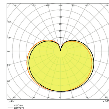
P CLAS A 40 FR 5.2 W/2700K E27
