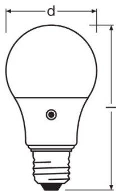
P CLAS A 40 FR 5.2 W/2700K E27
