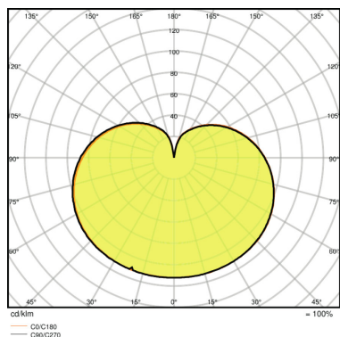
P CLAS A 60 FR 9 W/2700K E27
