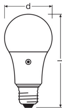
P CLAS A 60 FR 9 W/2700K E27, P CLAS A 75 FR 11 W/2700K E27
