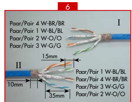
F/FTP - S/FTP
