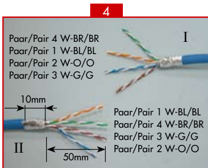
F/UTP - SF/UTP
