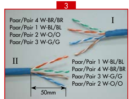
U/UTP
