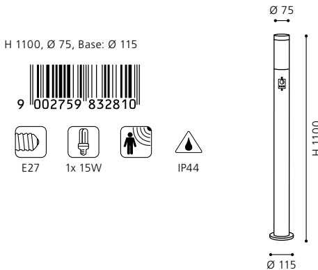
floor luminaire; stainless steel, stainless steel / plastic, white Stehleuchte; Edelstahl, edelstahl / Kunststoff, weiss lampadaire; acier inoxydable, acier inoxydable / plastique, blanc
