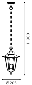
pendant luminaire; cast aluminium, black / glass, clear Hängeleuchte; Aluguss, schwarz / Glas, klar luminaire suspension; aluminium moulé, noir / verre, clair
