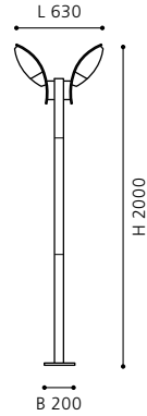
floor luminaire; cast aluminium, anthracite / plastic, white Stehleuchte; Aluguss, anthrazit / Kunststoff, weiss lampadaire; aluminium moulé, anthracite / plastique, blanc
