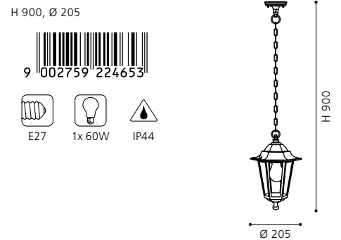
pendant luminaire; cast aluminium, white / glass, clear Hängeleuchte; Aluguss, weiss / Glas, klar luminaire suspension; aluminium moulé, blanc / verre, clair
