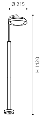
floor luminaire; stainless steel, stainless steel / plastic, white Stehleuchte; Edelstahl, edelstahl / Kunststoff, weiss lampadaire; acier inoxydable, acier inoxydable / plastique, blanc
