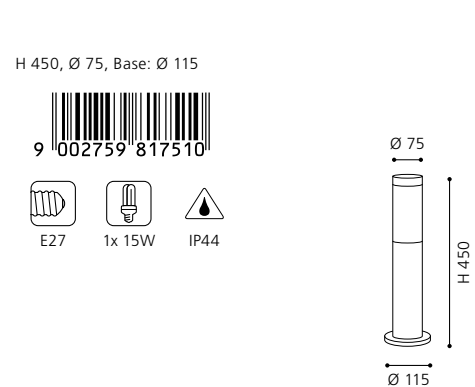
floor luminaire; stainless steel, stainless steel / plastic, white Stehleuchte; Edelstahl, edelstahl / Kunststoff, weiss lampadaire; acier inoxydable, acier inoxydable / plastique, blanc
