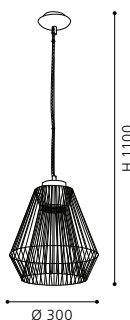
pendant luminaire; steel, white, cable black and white Hängeleuchte; Stahl, weiss, Kabel schwarz-weiß luminaire suspension; acier, blanc, câble noir et blanc
