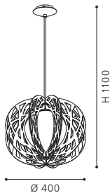
pendant luminaire; steel, satin nickel / plastic, glass, black- transparent, white Hängeleuchte; Stahl, nickel-matt / Kunststoff, Glas, schwarz-transparent, weiss luminaire suspension; acier, nickel mat / plastique, verre, noir- transparent, blanc
