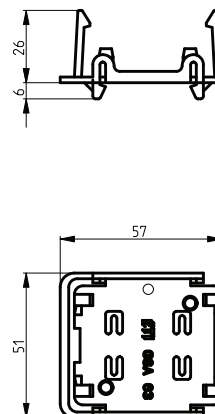
piesa din plastic pentru montaj GSA 63
