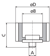
VD II pentru soclu siguranță E27
