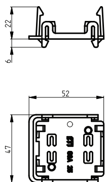
piesa din plastic pentru montaj GSA 25
