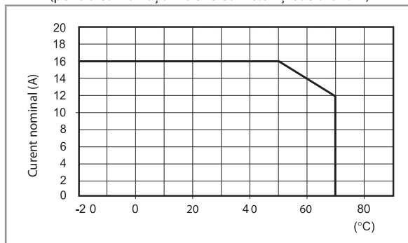
L 97 - Curent nominal vs. temperatura ambiantă (pentru combinația între releul 46.61 și soclul 97.11)
