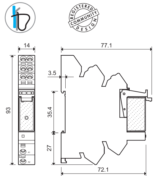
Tipurile 38.11 38.41 38.62 Terminal cu prindere rapidă
