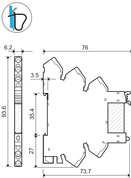
Tipurile 38.61/38.61.3 38.91/38.91.3 Terminal cu prindere rapidă
