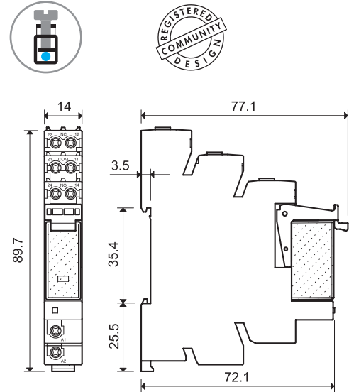
Tipurile 38.01 38.31 38.52 Terminal cu șurub
