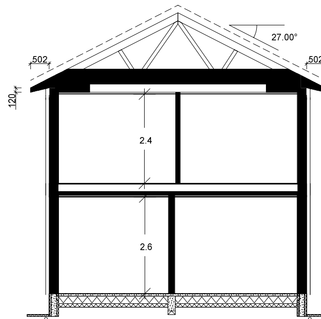
SNITT B-B
