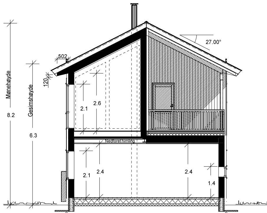
SNITT A-A
