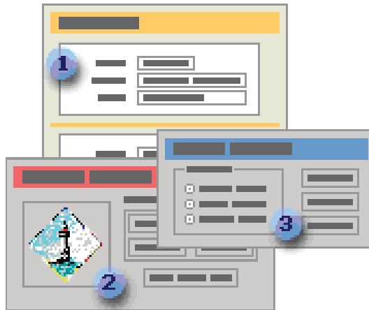
Gambar 11.36. Jenis-jenis form.
