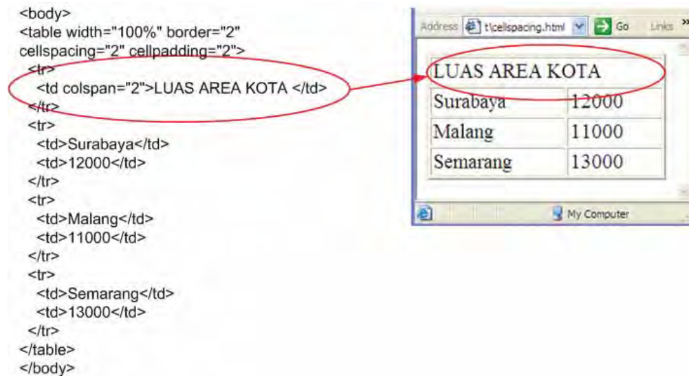
Gambar 13.35. Colspan.
