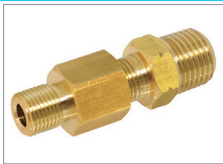
中間ニップル G1/8(外) × R1/4(外)
