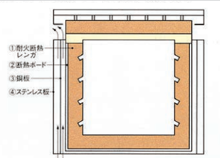
DAM シリーズの構造図
