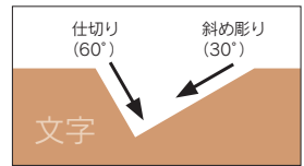
図c 片切り彫り 切り出して仕切り(約60°)を入れ、逆方向から丸刀などで斜め(約30°)に彫る。
