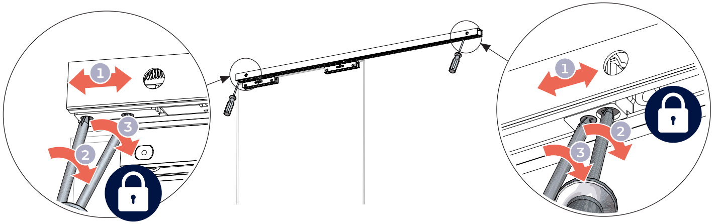
Porte simple / Single door
