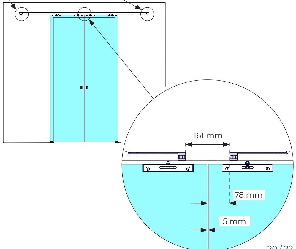
Porte double / Double door
