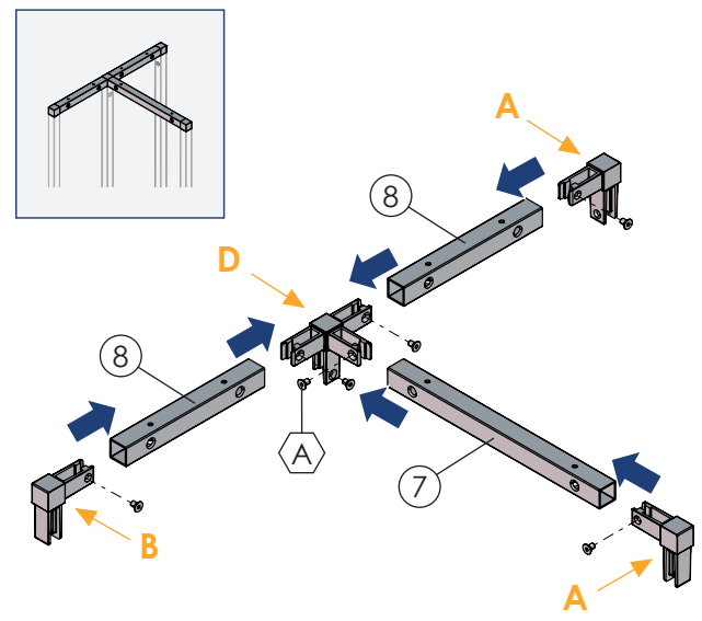
Partie haute / Upper part
