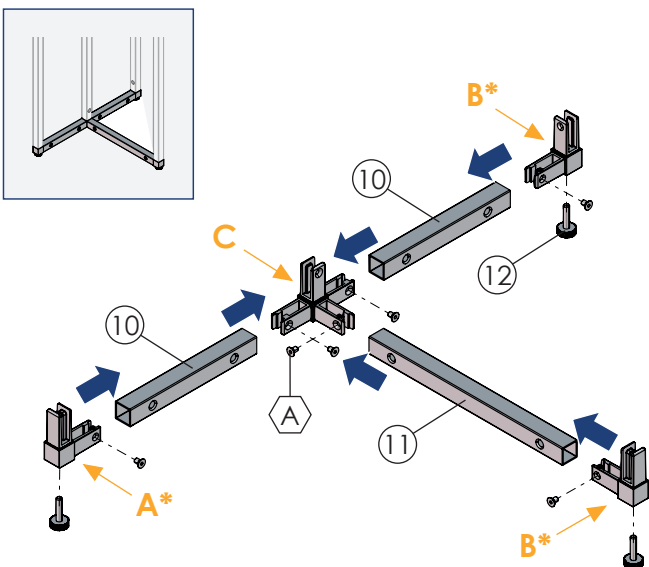
Partie basse / Lower part
