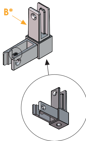
Angle B* (pour pied) / Corner B* (for leg)
