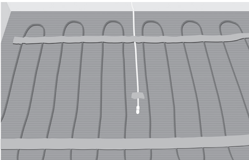
Kuva 9. Johtoputken/tunnistimen asettaminen kahden kaapelin väliin
