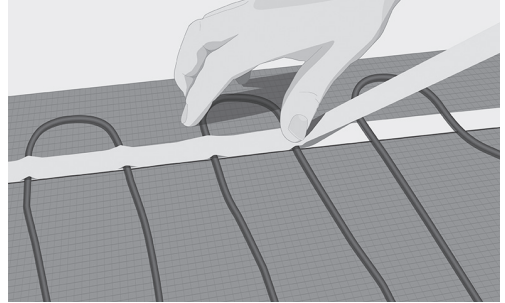
Kuva 8. Kiinnitä kaapeli maalarinteipillä
