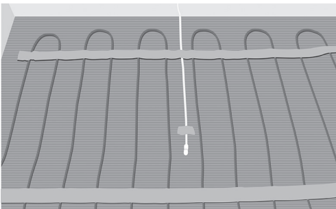
Fig. 9. Plasser ledningsrør/føleren mellom to kabler
