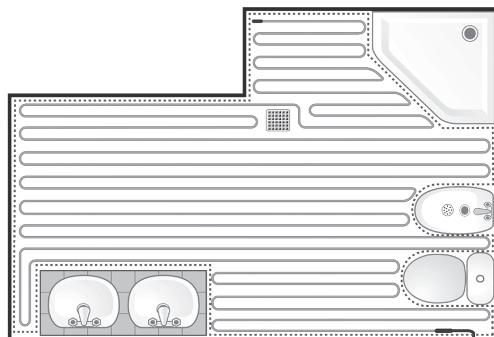
Рис. 1. Чертеж пола
