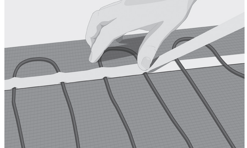
Fig. 8. Lås fast kabelen med maskeringstape
