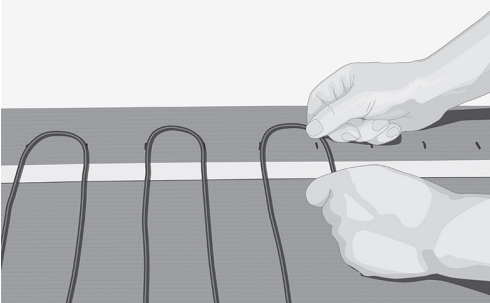
Fig. 7. Legg ut kabelen i henhold til c-c-merkingen
