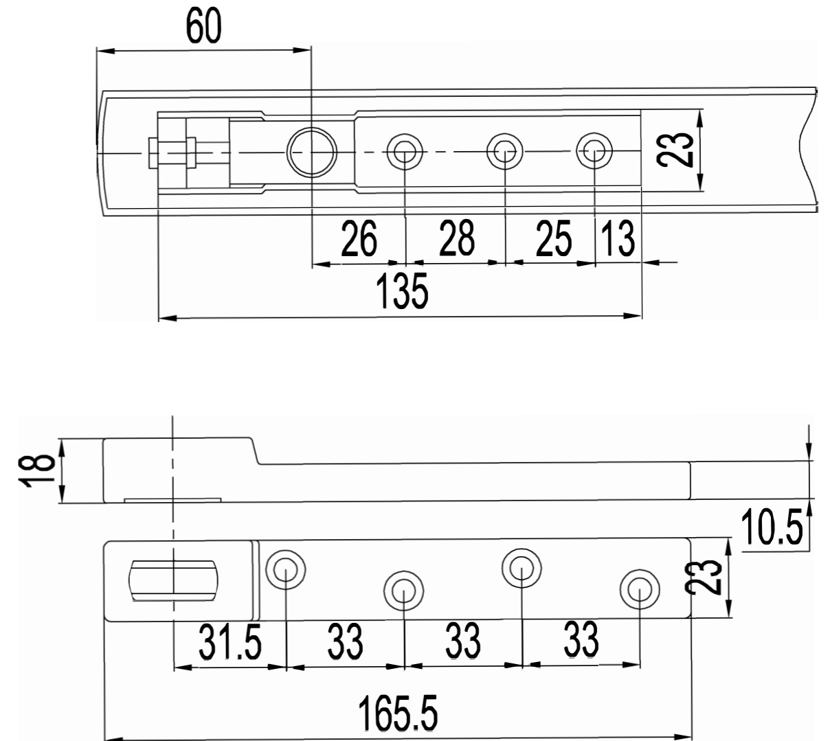
Top pivot (Door side)
