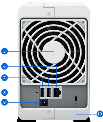
DS223j (Rückseite)
