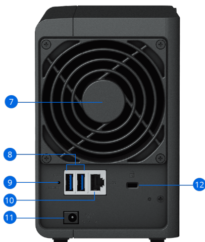
DS223 (Rückseite)
