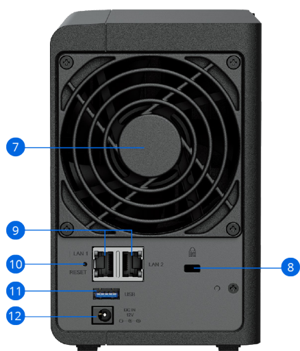
DS224+ (arrière)
