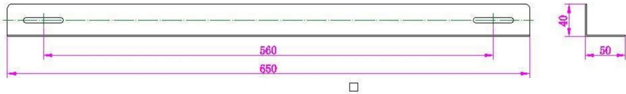
650深L角铁
