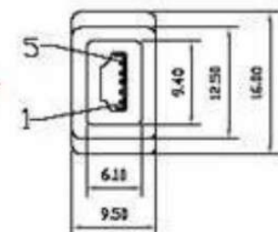
MINI USB 5P MALE
