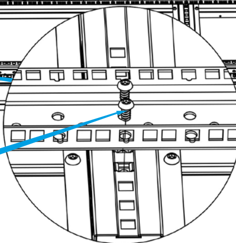
Allen head bolt M6 (part U)
