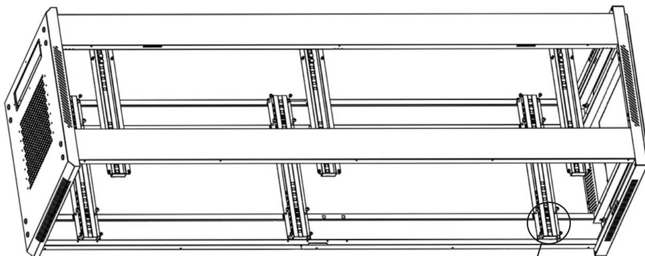
Allen head bolt M6 (item U)
