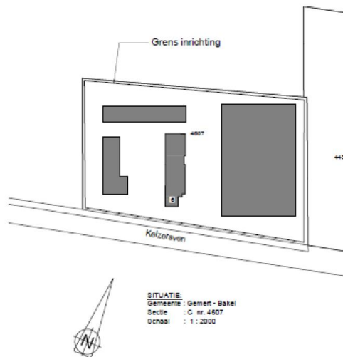
Afbeelding 3: Situering bebouwing beoogde situatie
