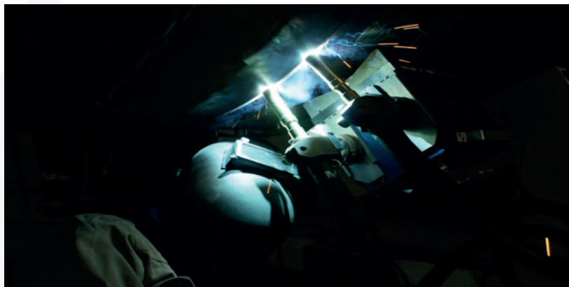
Veraweld in actie: lasrobot voor pijpleidingen. Onderscheidend product geproduceerd door Vermaat Technics in Rockanje.
