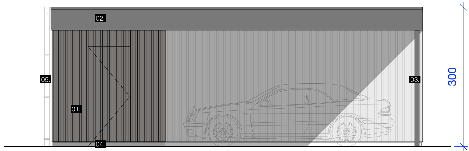
ZIJGEVEL
