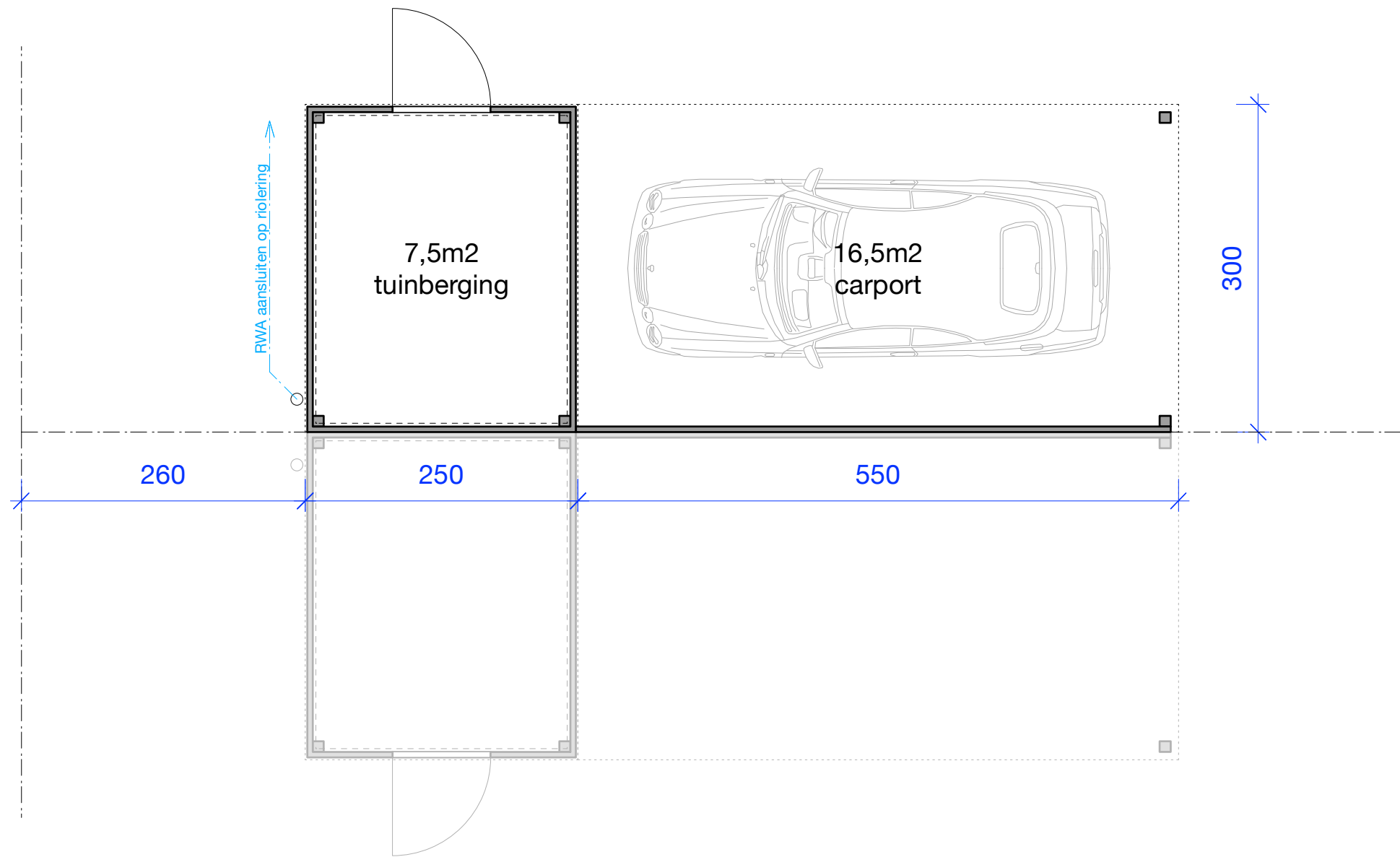
GRONDPLAN
