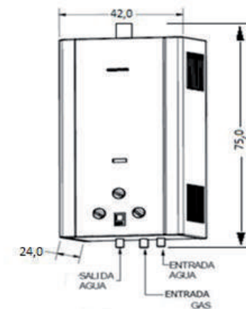
Dimensiones en cm
