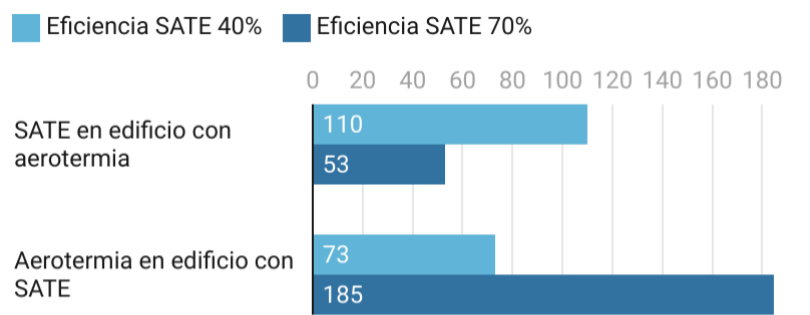
Figura 14. Plazo de amortización (años) para intervenciones de aerotermia con SATE previo vs SATE con aerotermia previa
