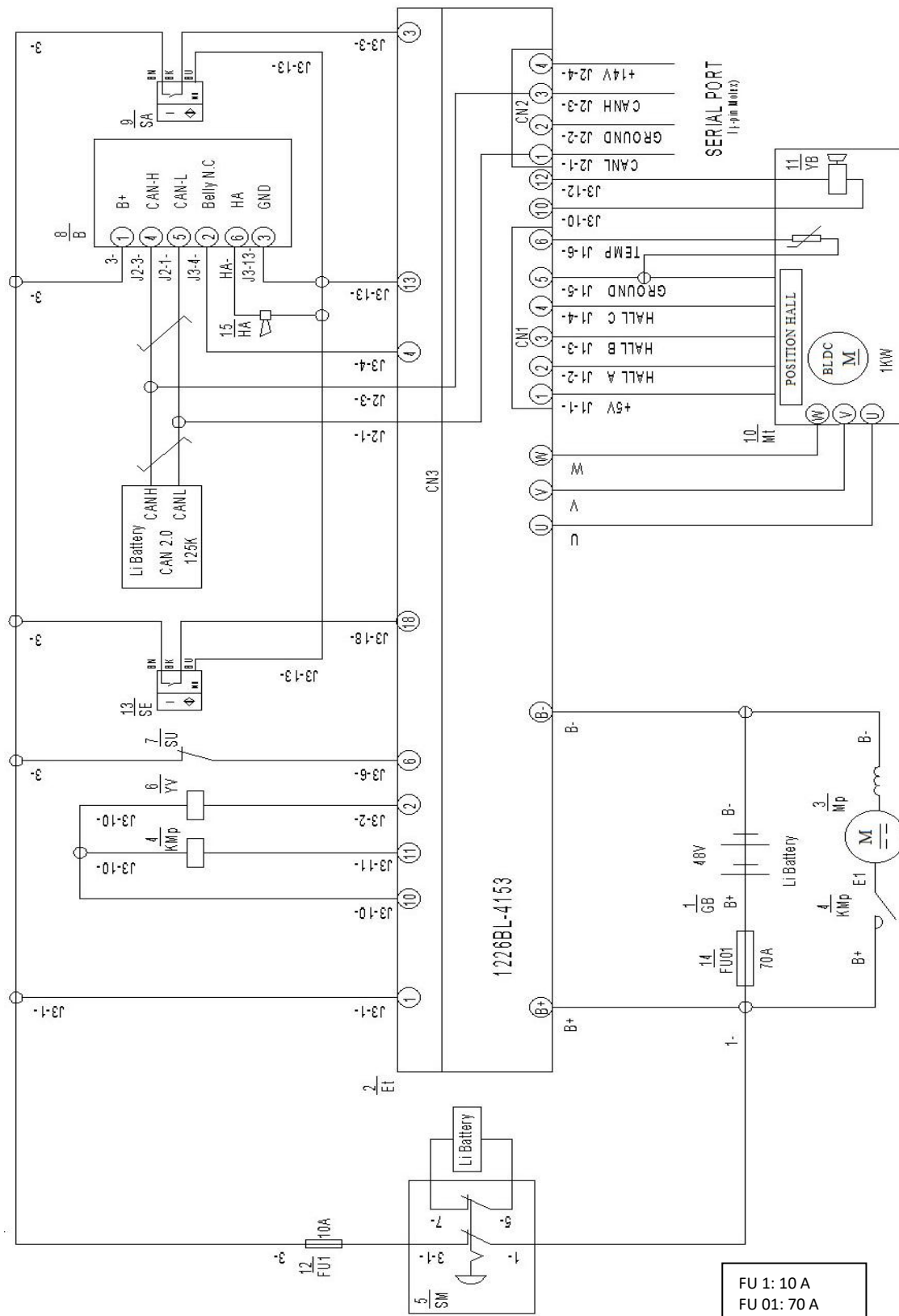
Figura 18: Schema elettrico EZY-20
