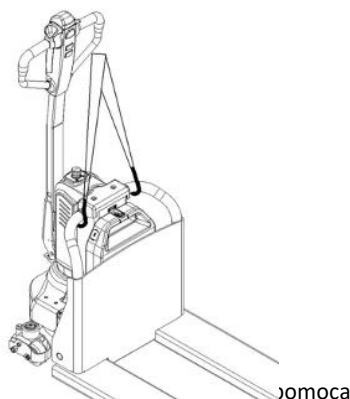
Ilustracja 53: Mocowanie za pomocą dźwigu
