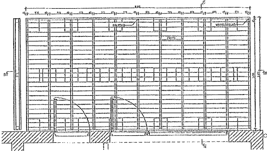
PLAN SKALA 1:20 Trädäck tvåbostadshus
