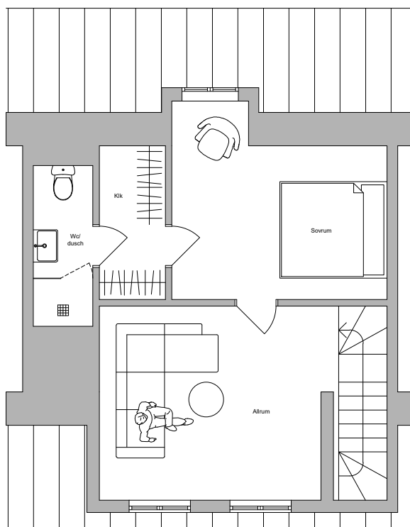
Bostad 5 Vindsplan 36 kvm Skala 1:100
