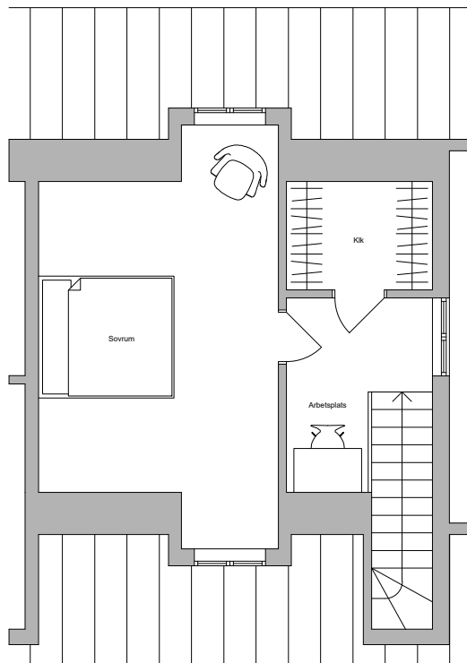
Bostad 6 Vindsplan 25,5 kvm Skala 1:100
