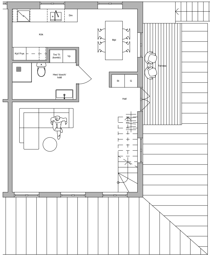
Bostad 6 Plan 2 49,5 kvm Skala 1:100
