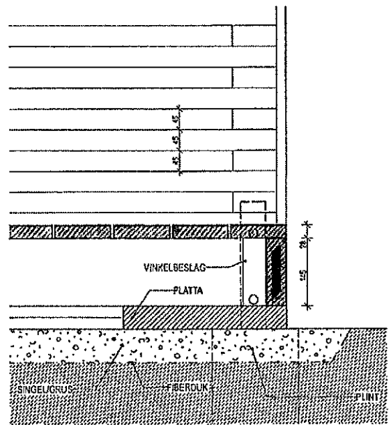
DETALJ D1 SKALA 1:5
