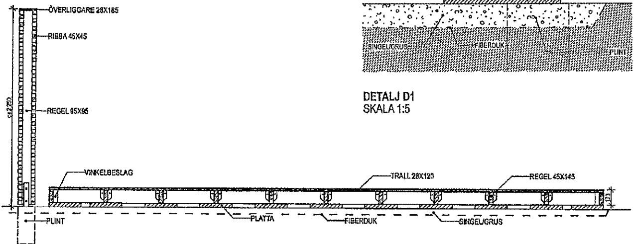
SEKTION A-A SKALA 1:20
