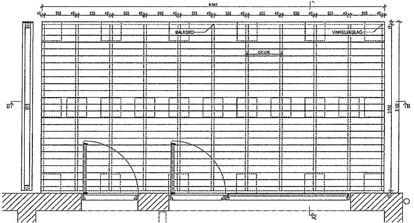
PLAN SKALA 1:20
