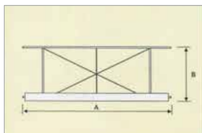
Baranda zócalo
