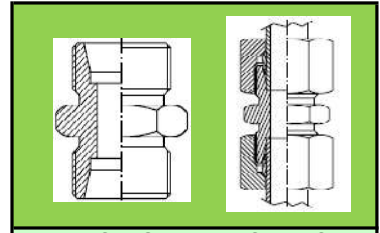
UNION IGUAL TUBO-TUBO
