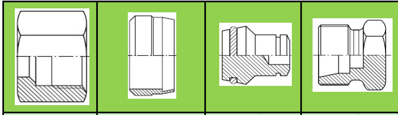
TUERCA BICONO TAPON BICONO TAPON MACHO
