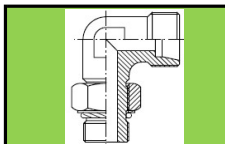
CODO ORIENT.BSPP
