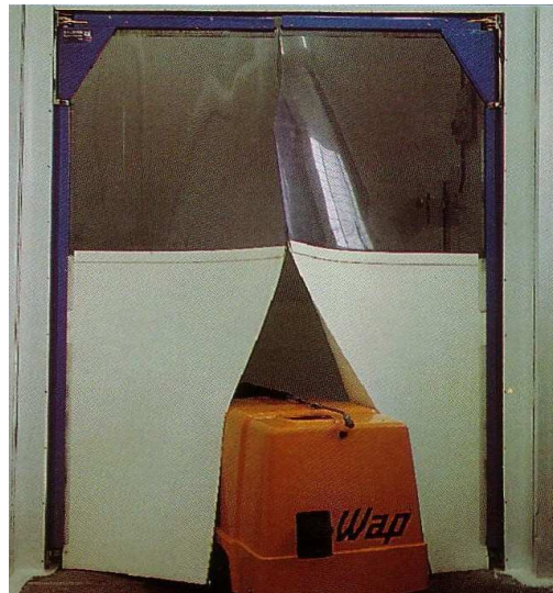
Puerta batiente, acabados en esmalte sintético azul y hojas de PVC en versión mixta blanca.
