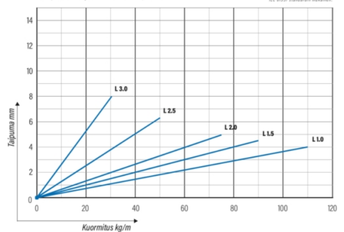
KRA/KRB 90 | LEVEYDET 100, 200
