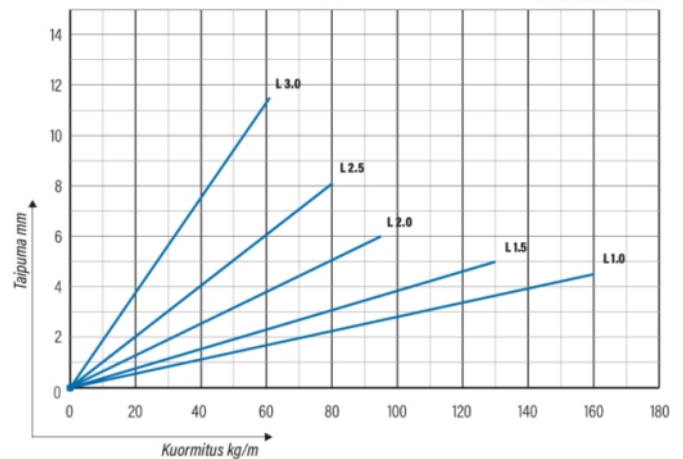
KRA/KRB 90 | LEVEYDET 400, 500, 600
