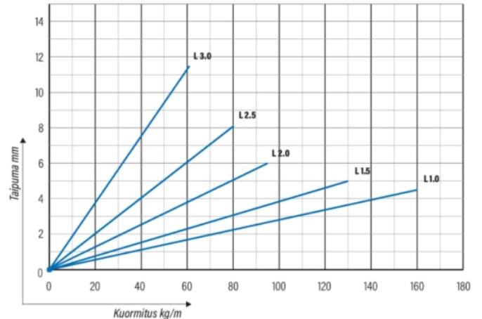
KRA/KRB 60 | LEVEYDET 400, 500, 600
