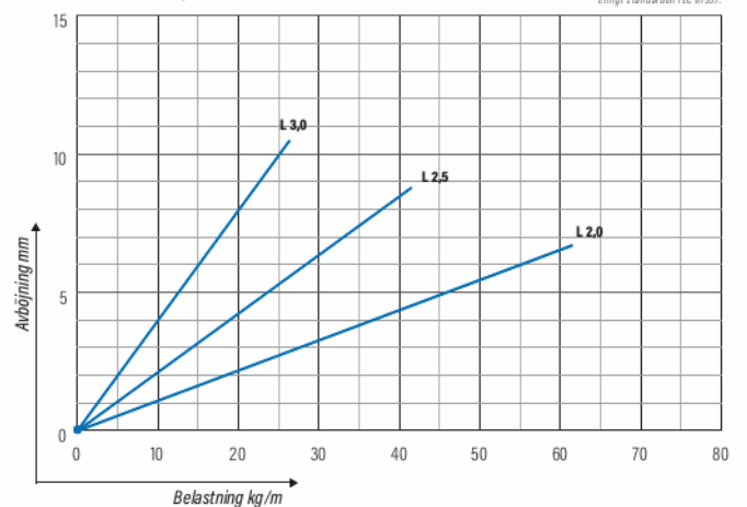
KRA/KRB 40 | BREDD 100, 200
