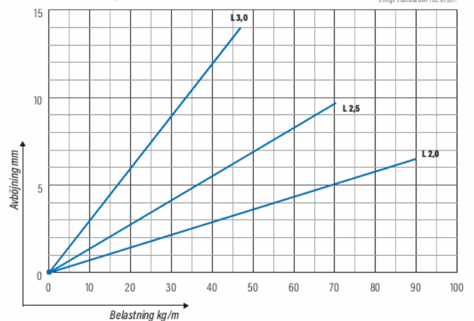
KRA/KRB 40 | BREDD 400, 500, 600
