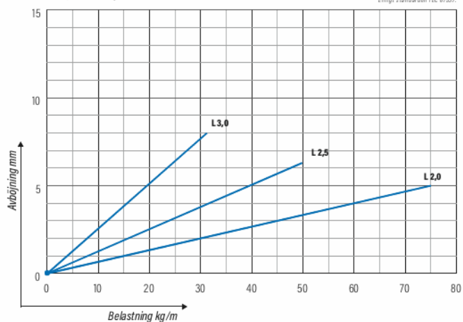
KRA/KRB 60 | BREDD 100, 200
