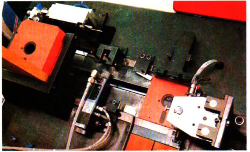
▲ Kapaklar kapanıyor: Son katlayıcı kabı kapatıyor.
