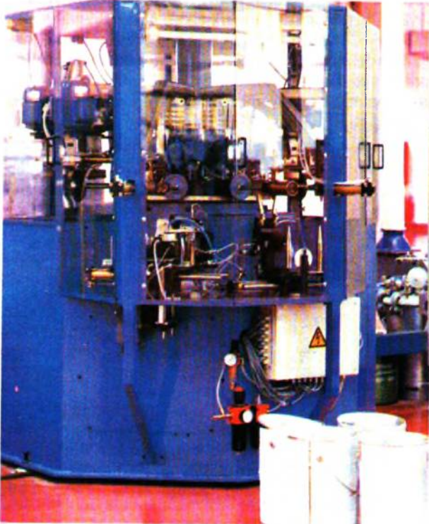
► Yuvarlak vuruş makinesi, tabaka yüzeylerinin düzeltilmesini sağlar.
